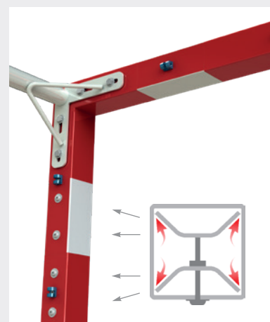
Focus fixation PostLock®, arceau et maillon de filet
